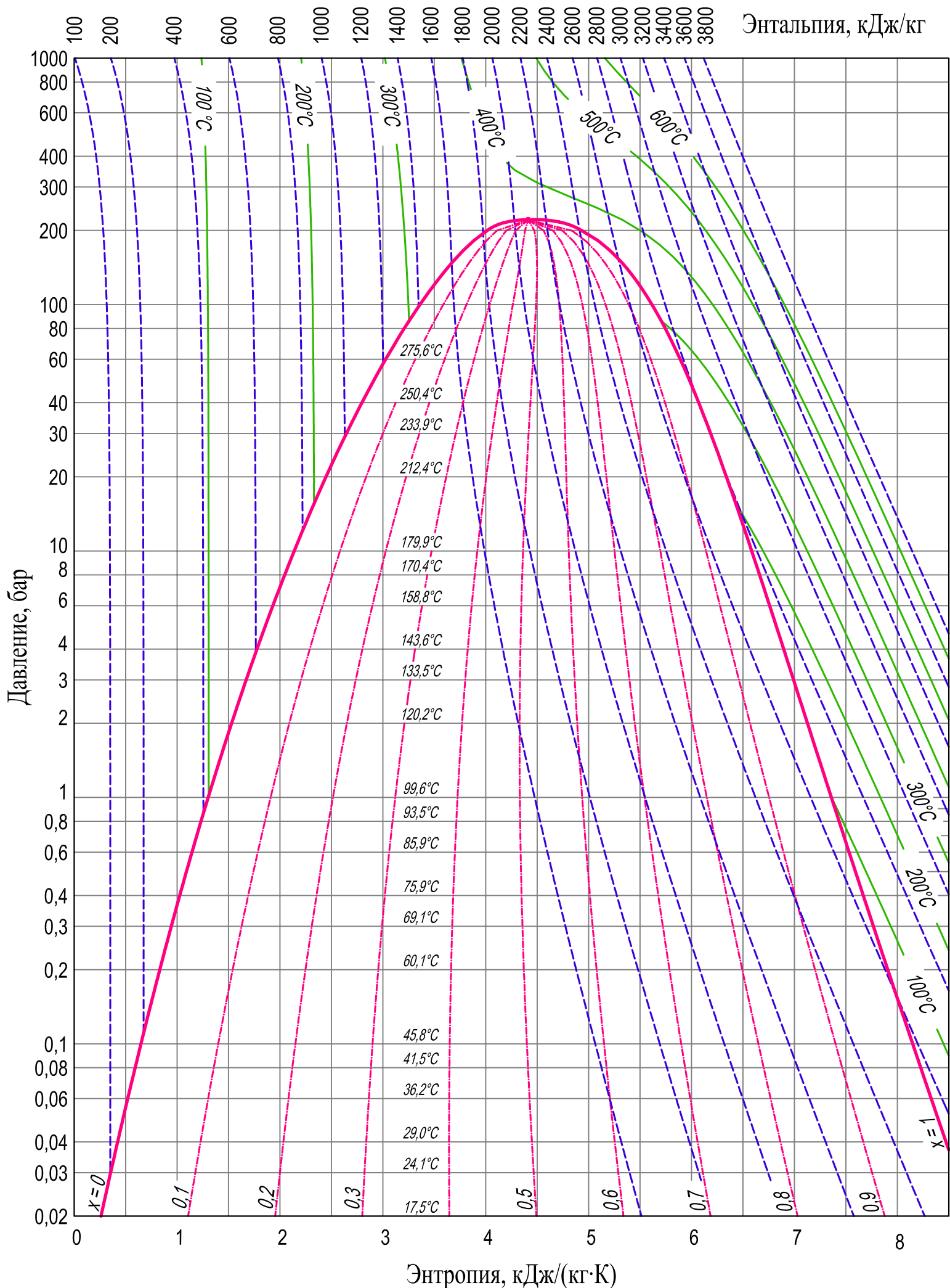
P - s -диаграмма воды и водяного пара
