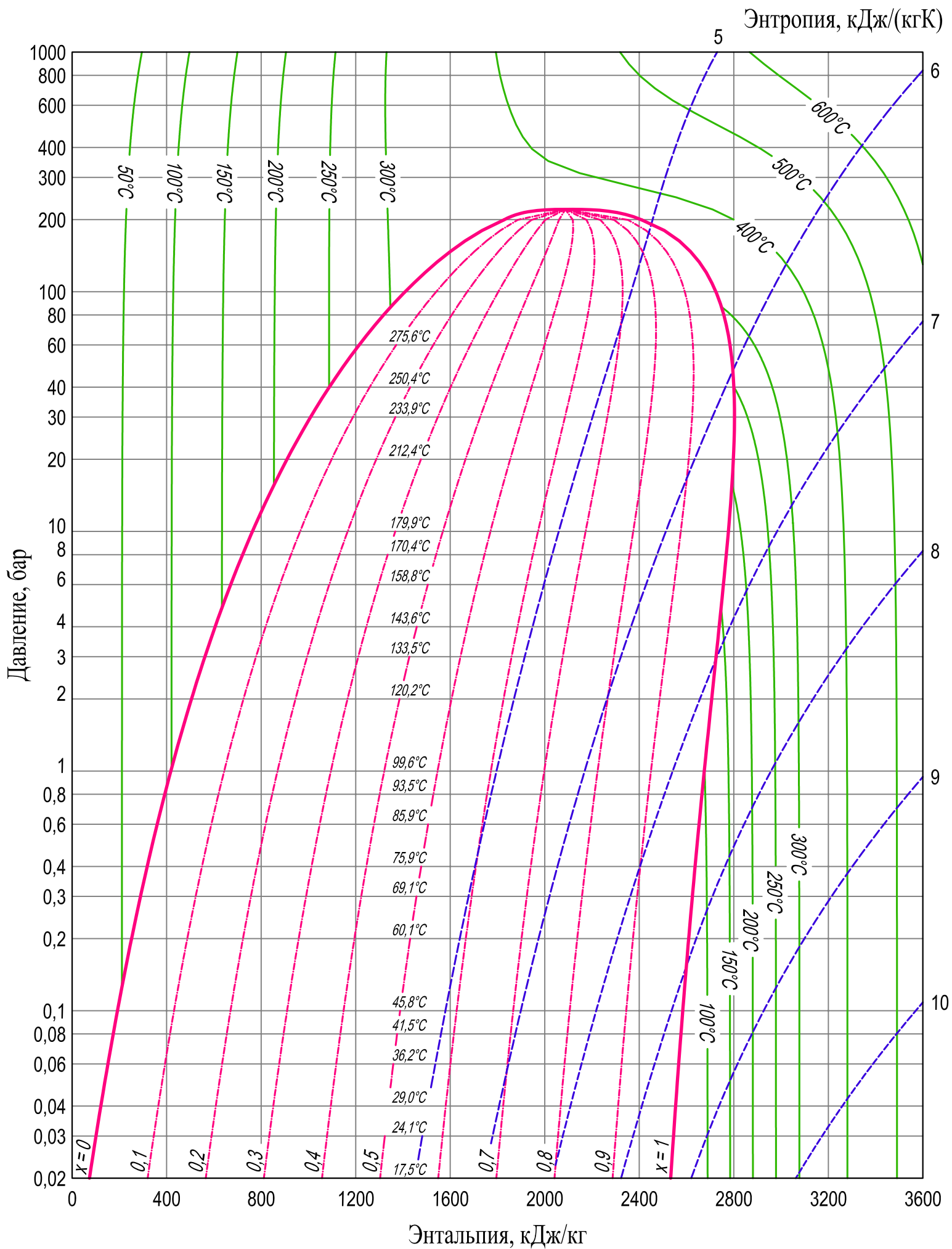
P-h-диаграмма воды и водяного пара
